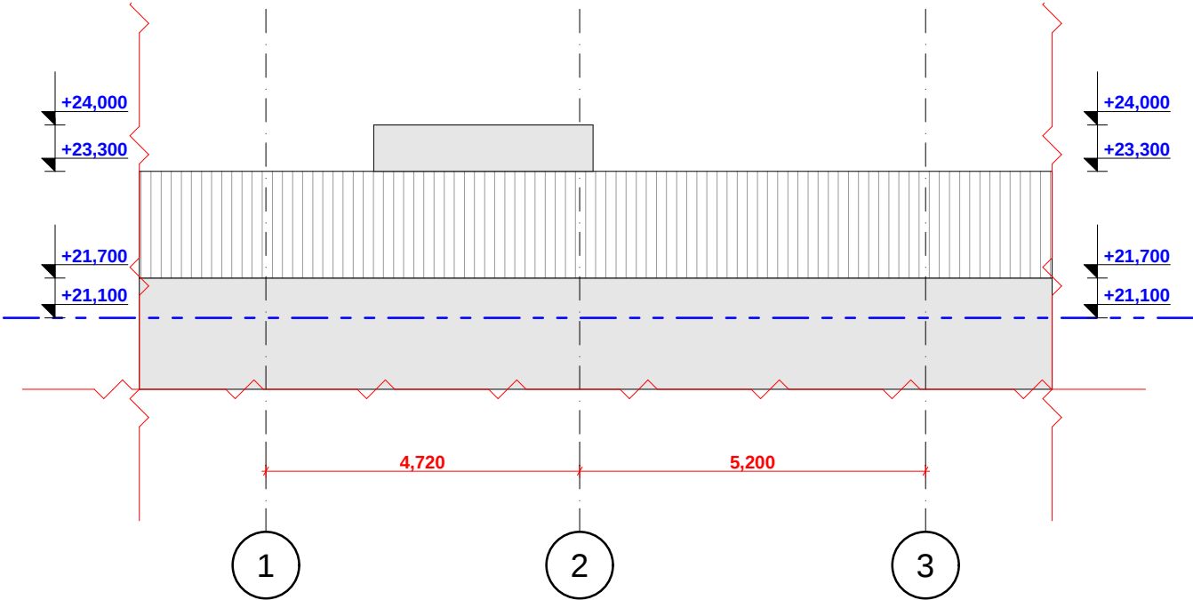
a r sebu l i fasad i 1-3 ReRZebSi m. 1:100
