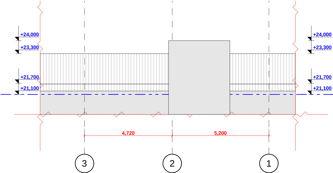
sap r oeq t o fasad i 3-1 ReRZebSi m. 1:100
