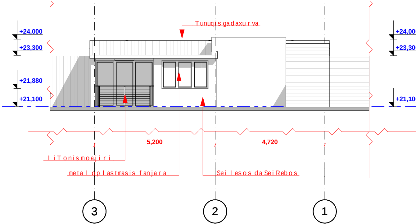
sap r oeq t o fasad i 3-1 ReRZebSi m. 1:100
