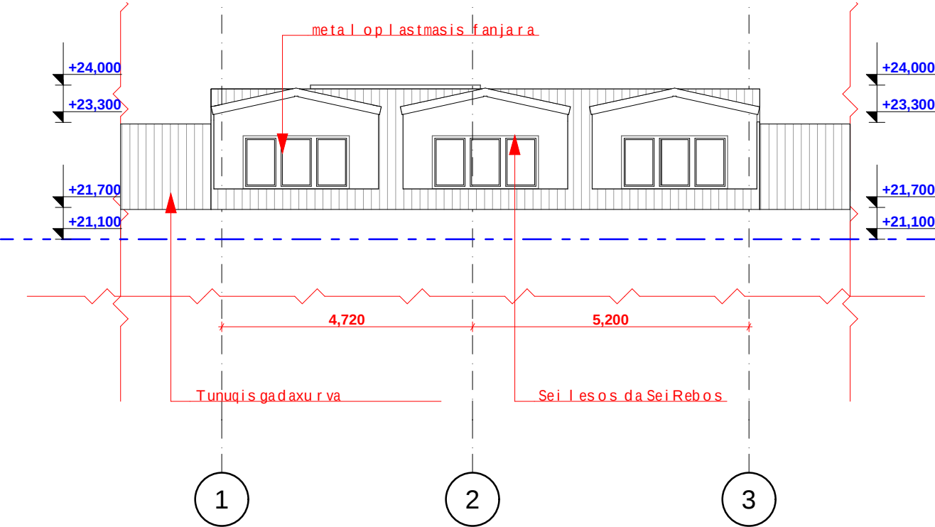
sap r oeq t o fasad i 1-3 ReRZebSi m. 1:100
